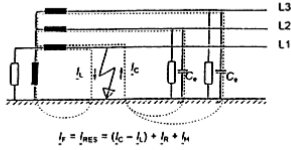
Şekil-4b Toprak teması kompanze edilmiş (rezonans topraklı) bir şebekede toprak hata akımı
