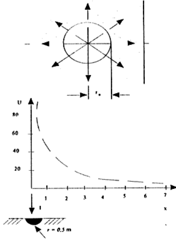
Şekil-T.5 Yarımküre topraklayıcıda akım ve potansiyel dağılımı
