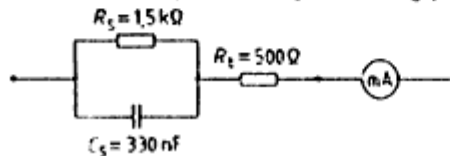
Şekil-10 100 Hz'in üzerindeki frekanslara sahip periyodik akımların ölçülmesi için bağlantı devresi
