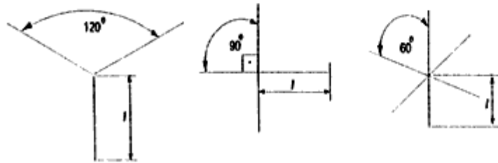
Şekil-T.8 Yıldız topraklayıcı çeşitleri
