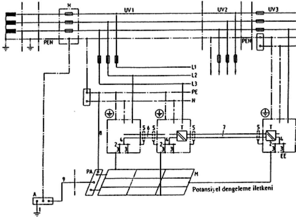
Şekil-27 Ayrı şebeke beslemesinin başka bir alt dağıtım panosundan beslenen ve ekranlı sinyal iletim hatlarıyla bağlanan uzaktaki bir son cihaza sahip iletişim tesisinin topraklamasına örnek (Not: Bu şekil mecburi olmayıp, yalnızca bir fikir vermek amacıyla taşınmaktadır.)
