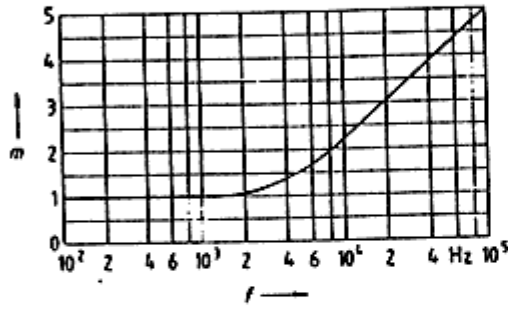
Şekil-Y.7 Frekansa f bağılı olarak frekans katsayısı m 'nin değişimi
