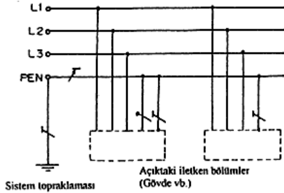
Şekil-5c TN-C Sistemi. Sistemin tamamında nötr ve koruma fonksiyonları, tek iletkende birleştirilmiştir
