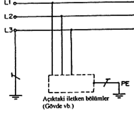
Sistem topraklaması
