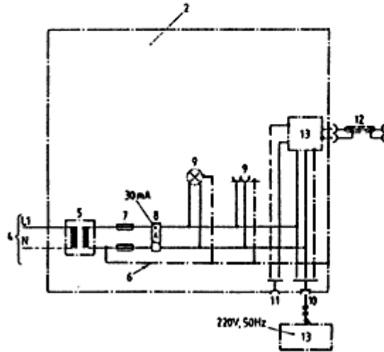
Şekil-30 Madde 28-d2'de belirtilen, bir fazlı alternatif akıma bağlı, ayırma transformatörlü, aşırı akım ve hata akımı koruma düzenleri ve potansiyel dengelemesi bulunan bir sinyal iletim tesisine örnek (Not: Bu şekil mecburi olmayıp, yalnızca bir fikir vermek amacıyla taşınmaktadır.)
