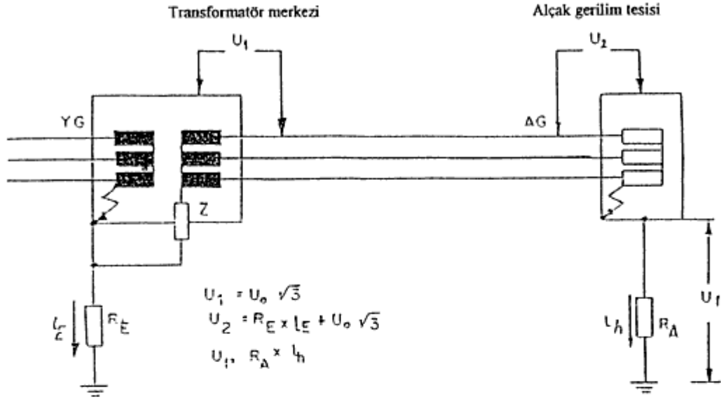
AG sistemlerinde ilk arızanın oluşması
