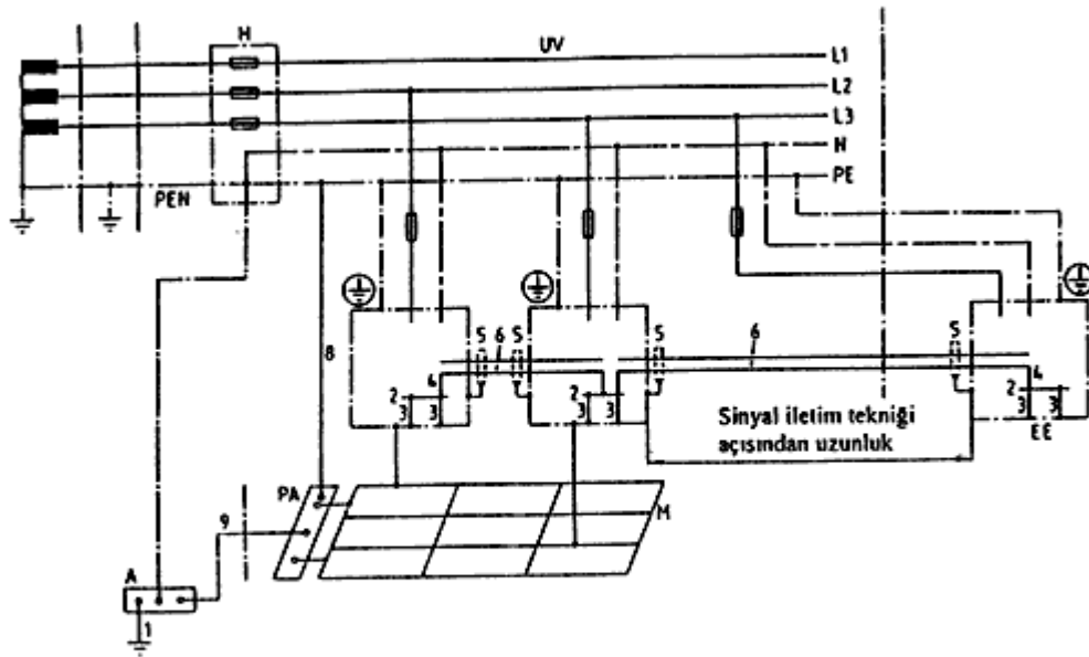
Şekil-25 Aynı alt dağıtım panosundan beslenen uzaktaki bir son cihaza sahip iletişim tesislerinin topraklamasına örnek (Not: Bu şekil mecburi olmayıp, yalnızca bir fikir vermek amacıyla taşınmıştır.)
