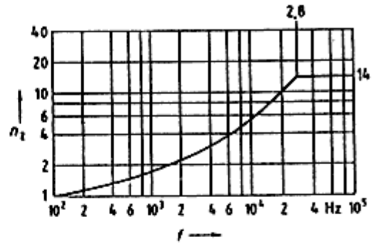
Şekil-Y.6 Frekansa/bağılı olarak frekans katsayısı n_2 'nin değişimi
