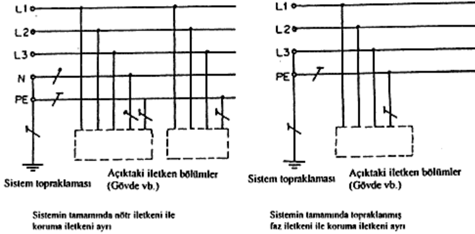
Şekil-5a TN-S Sistemi
