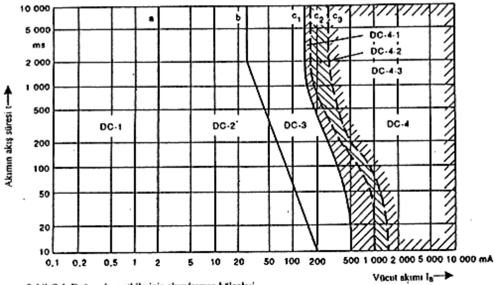
Şekil-C.4 Doğru akım etkilerinin akım/zaman bölgeleri
