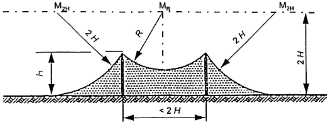
Şekil-II.2 İki koruma teli
