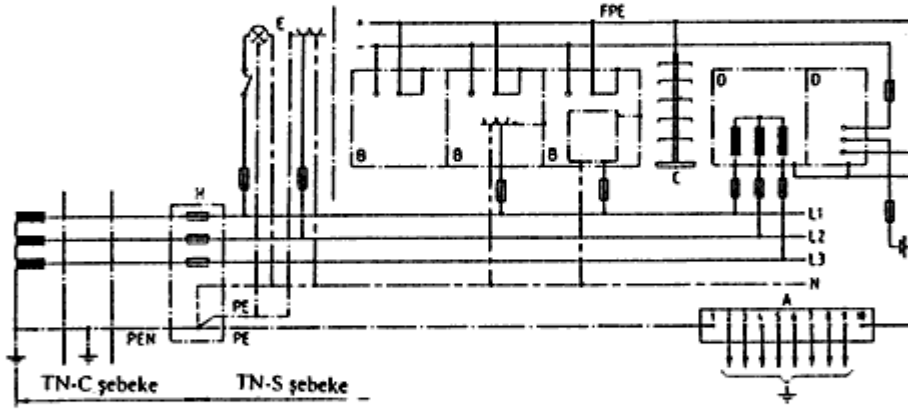
Şekil-18 Madde 21-b3'de belirtilen bir iletişim tesisinin fonksiyon ve koruma topraklamasına örnek (Not: Bu şekil mecburi olmayıp, yalnızca bir fikir vermek amacıyla taşınmaktadır.)
