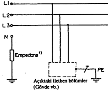
Sistem topraklaması
