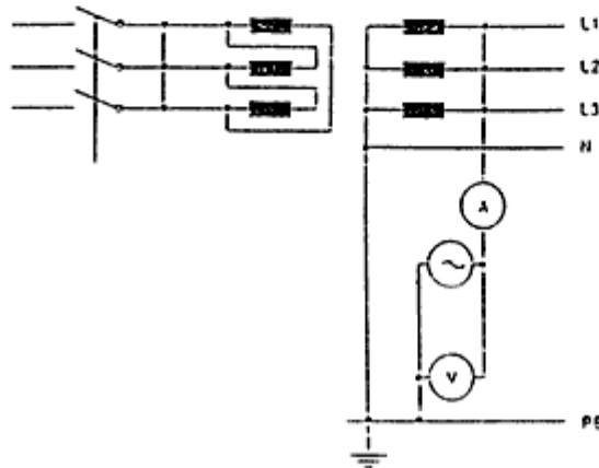
Şekil-N.3 Arıza çevrim (halka) empedansının ayrı bir besleme yardımı ile ölçülmesi deneyi
