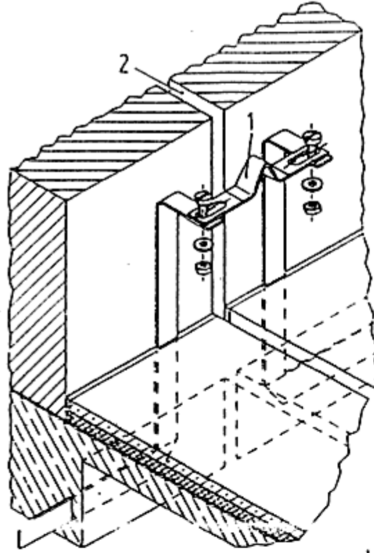
Şekil-L.4 İnşaatların içinde, esnek bağlantı ile hareket aralıklarının köprülenmesine örnek
