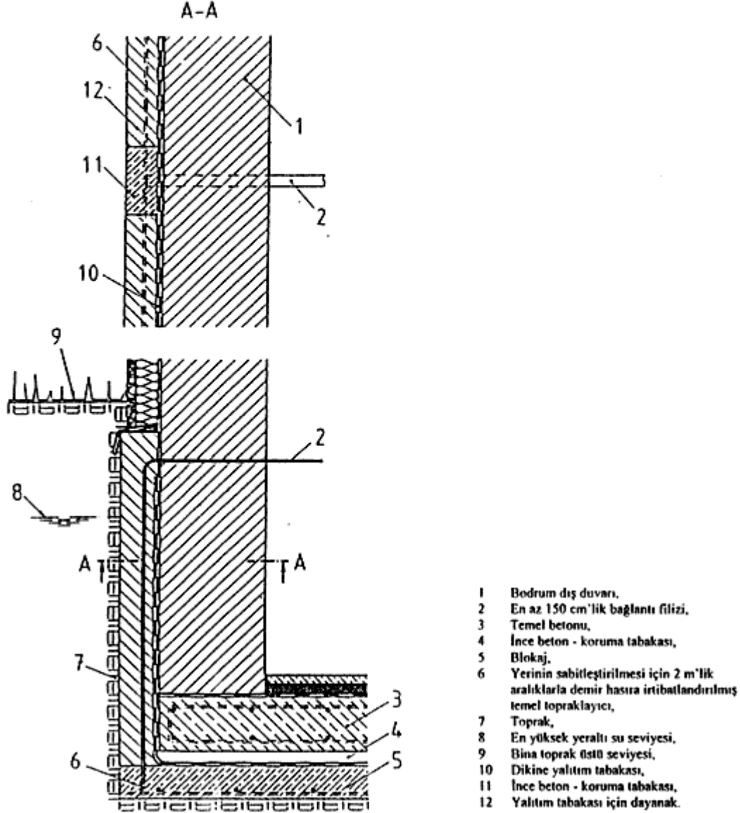
Şekil-L.7 Bina temeli yalıtım malzemesi içinde kalan temel topraklayıcısının yerleştirilmesine örnek
