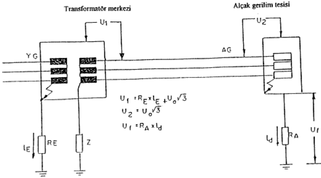
AG sisteminde ilk arızanın oluşması
