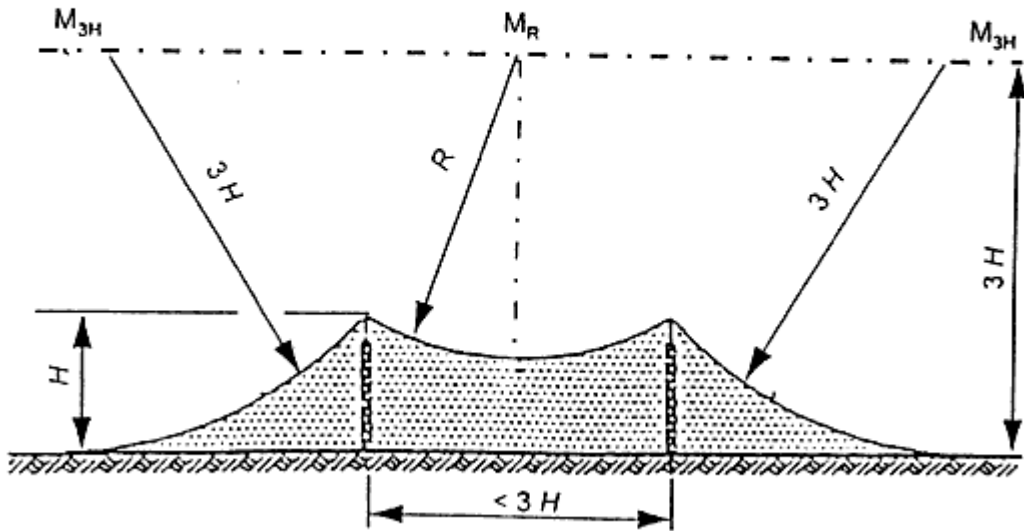
Şekil-II.4 İki yıldırım yakalama çubuğu
