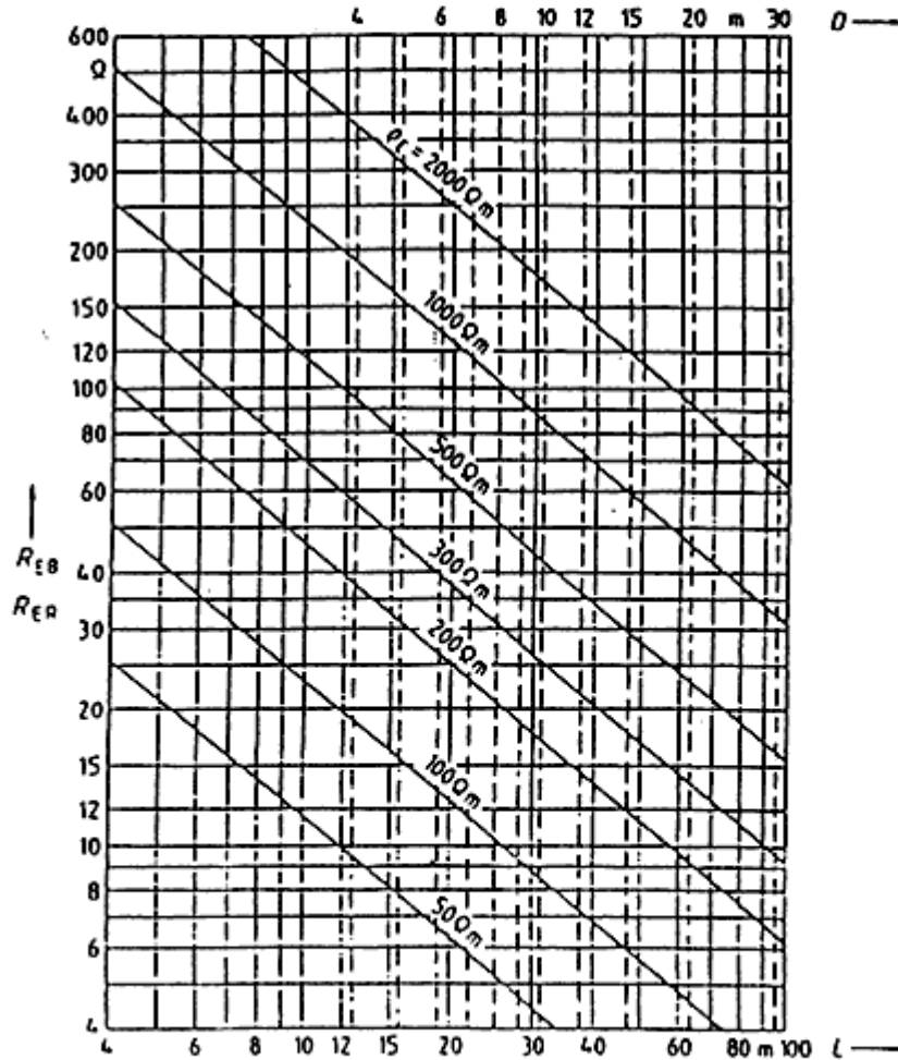
Őekil-K.1 Homojen toprak ierisinde halka Őeklinde veya d z olarak yerleřtirilmiř (Őeritten, yuvarlak malzemeden veya  rg tl  iletkenlerden yapılmıř) yatay topraklayıcıların yayılma direnci
