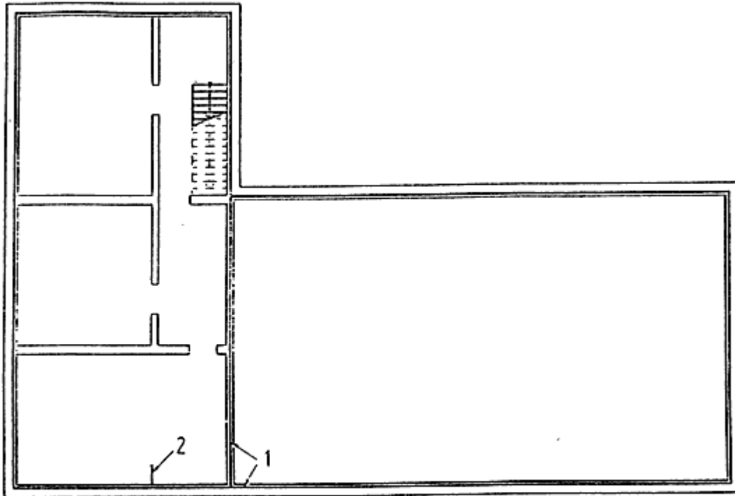
Şekil-1.2 Bitişik nizam evlerde temel topraklıyıcının yerleştirilmesine örnek
