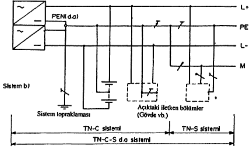
Şekil-5h TN-C-S Doğru akım sistemi
