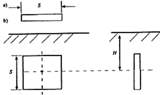
Şekil-T.12 Kare şeklindeki levha topraklayıcı
