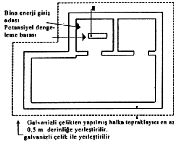
Şekil-T.10 Halka (ring) topraklayıcı
