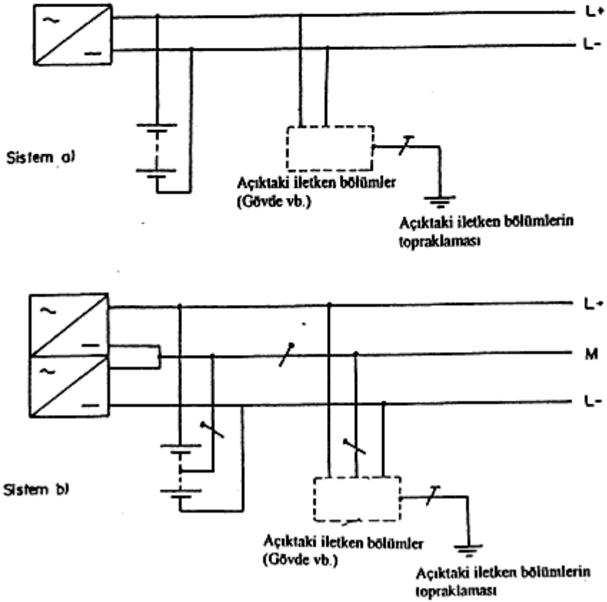
Şekil-5j TT Doğru akım sistemi
