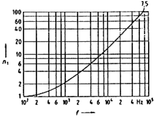
Şekil-Y.5 Frekansa/bağılı olarak frekans katsayısı n_1 'in değişimi
