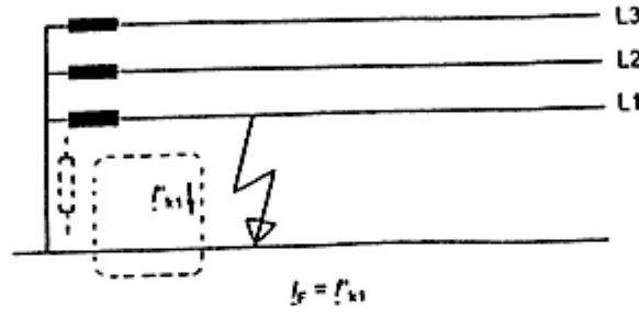
Şekil-4c Yıldız noktası, değeri düşük bir empedans üzerinden topraklanmış bir şebekede toprak hata akımı
