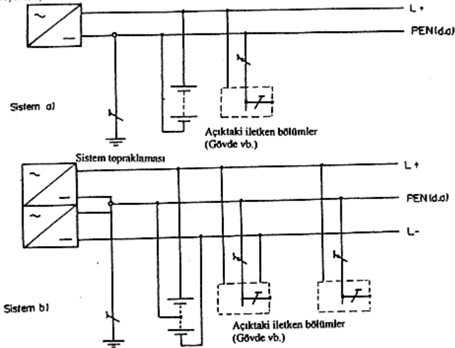
Şekil-5g TN-C Doğru akım sistemi
