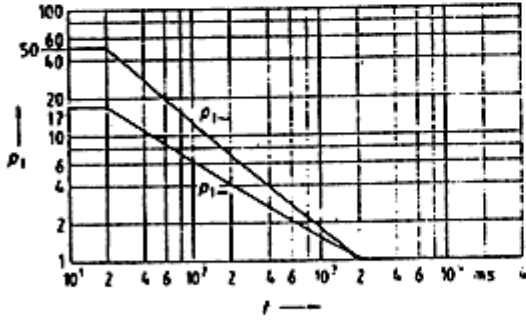
Şekil-Y.8 Etki süresine t bağılı olarak kısa süre katsayıları \rho_{1a} ve \rho_{1b} 'nin değişimi
