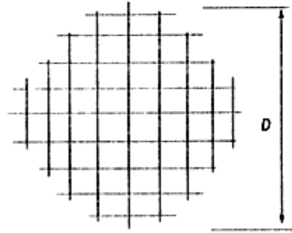
Şekil-T.9 Gözlü topraklayıcı
