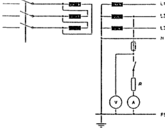
Şekil-N.2 Arıza çevrim (halka) empedansının gerilim düşümü yardımı ile ölçülmesi deneyi
