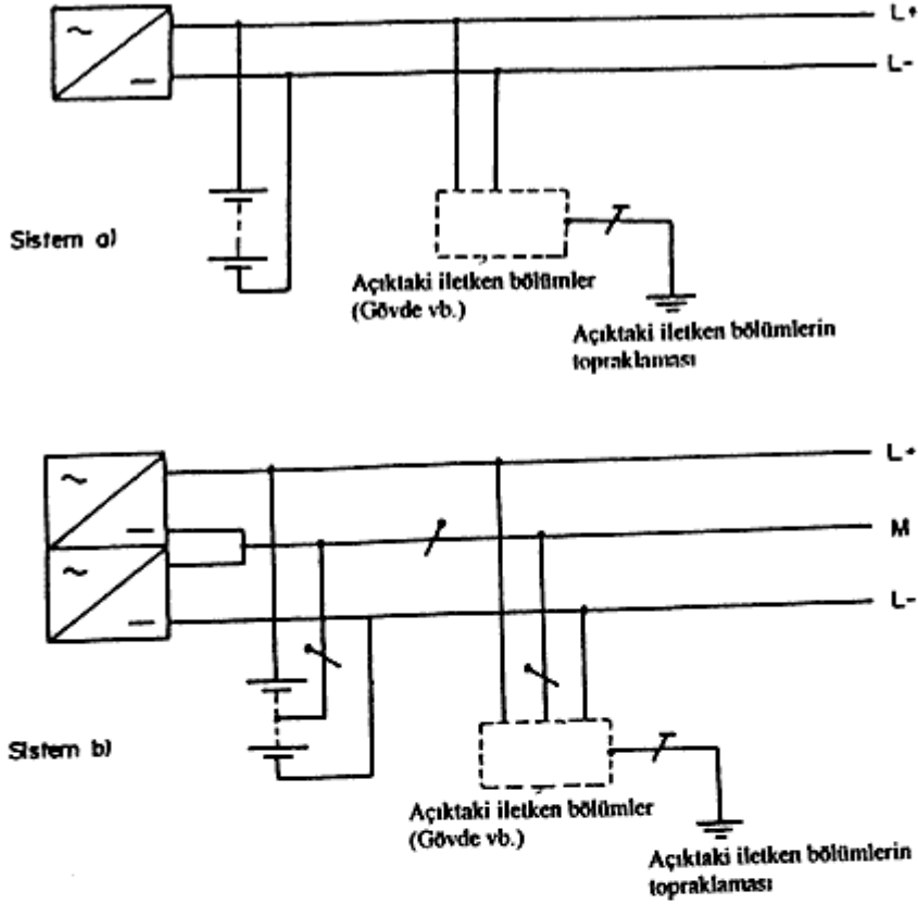
Şekil-5k IT Doğru akım sistemi
