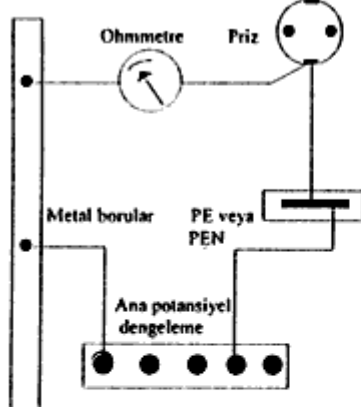
Şekil-8a Koruma iletkenlerinin bağlantısının ölçülmesi
