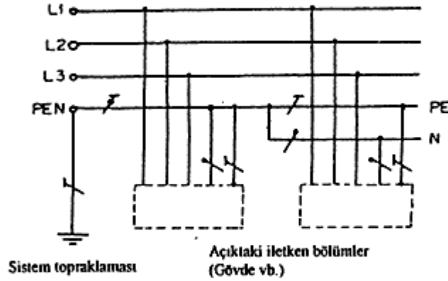
Şekil-5b TN-C-S Sistemi. Nötr iletkeni ve koruma iletkeni, sistemin bir bölümünde tek iletkende birleştirilmiştir
