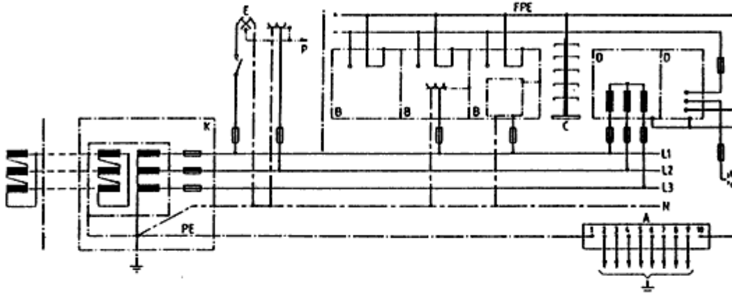
Şekil-16 Madde 21-b1'de belirtilen bir iletişim sisteminin fonksiyon ve koruma topraklamasına örnek (Not: Bu şekil mecburi olmayıp, yalnızca bir fikir vermek amacıyla taşımaktadır.)
