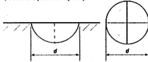
Şekil-T.14 Yarım küre şeklindeki topraklayıcı
