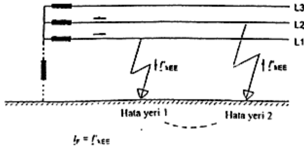
Şekil-4e Yıldız noktası yalıtılmış veya toprak teması kompanze edilmiş bir şebekede çift toprak teması akımı
