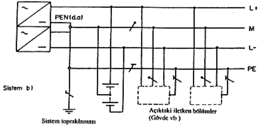
Şekil-5f TN-S Doğru akım sistemi
