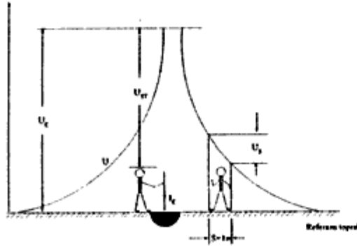
Şekil-T.2 Adım ( U_2 ), dokunma ( U_{S1} ) ve topraklama ( U_t ) gerilimlerinin şematik olarak gösterilmesi
