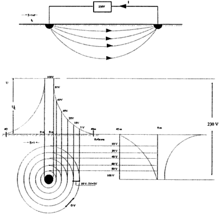
Şekil-T.4 Bir topraklayıcıda yayılma direncinin uzaklıkla değişimi
