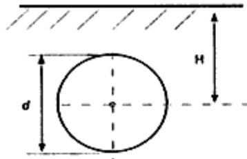
Şekil-T.13 Küre şeklindeki topraklayıcı
