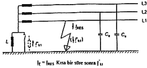
Şekil-4c Yıldız noktası, değeri düşük bir empedans üzerinden topraklanmış bir şebekede toprak hata akımı
