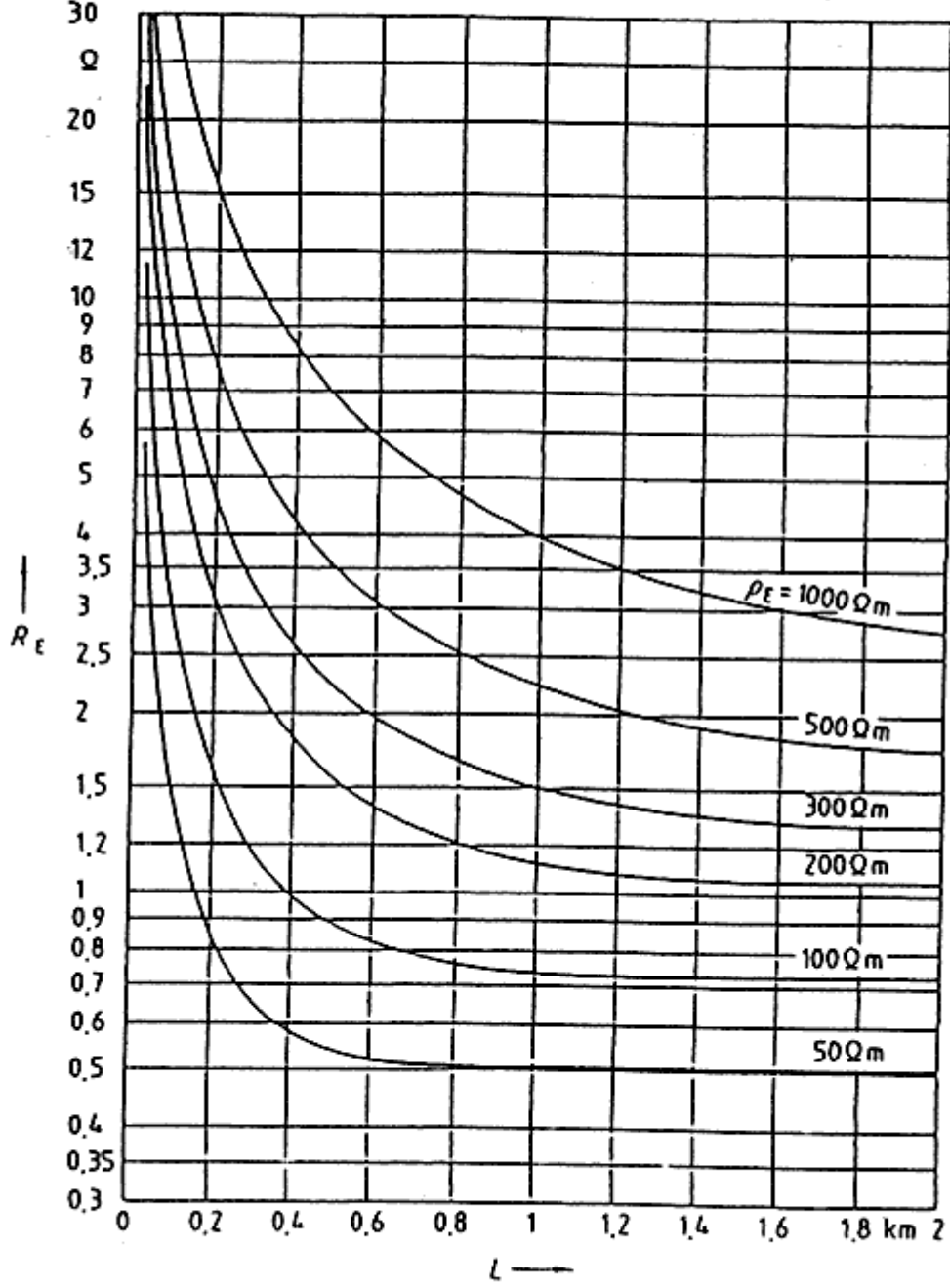
Şekil-K.3 Kablo boyuna ve toprak öz direncine bağlı olarak topraklayıcı etkisi olan kablonun yayılma direncinin tipik değerleri Muhtelif topraklayıcı tiplerine ilişkin hesaplama örnekleri Ek-T'de verilmiştir.
