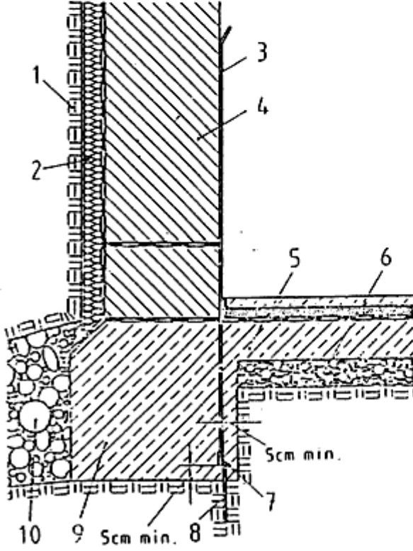
Şekil-L.5 Demir hasır olmayan (kuvvetlendirilmemiş) temel içinde temel topraklayıcının yerleştirilmesine örnek
