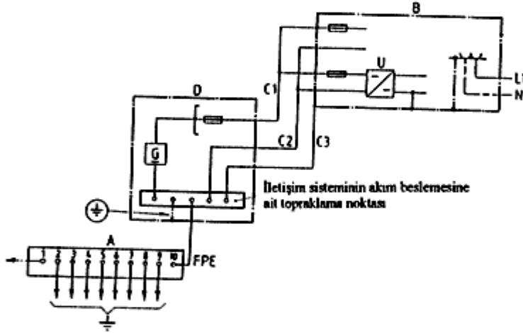
Şekil-15 İletişim sistemine ilişkin akım beslemesinin anma gerilimleri sınırlanmaksızın bir iletişim tesisi için ek topraklama ile yapılan işletme ve koruma topraklamasına örnek (Not: Bu şekil mecburi olmayıp, yalnızca bir fikir vermek amacıyla taşınmıştır.)
