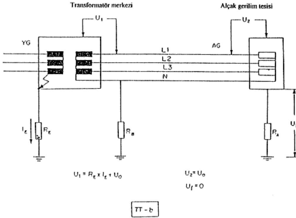
Şekil-9b TT sistemleri
