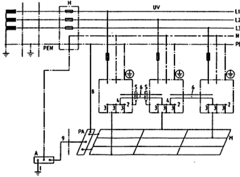
Şekil-24 Bir iletişim tesisinin santral merkezi ünitelerinin topraklamasına ve potansiyel dengelemesine örnek (Not: Bu şekil mecburi olmayıp, yalnızca bir fikir vermek amacıyla taşınmıştır.)
