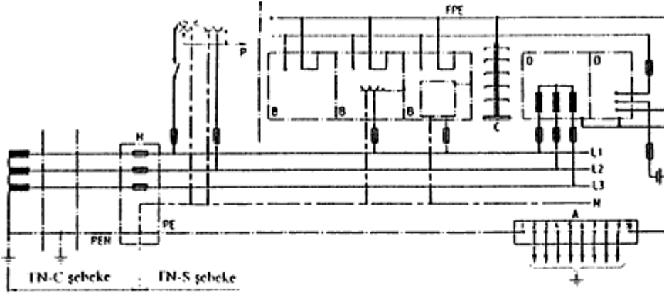
Şekil-17 Madde 21-b2'de belirtilen bir iletişim tesisinin fonksiyon ve koruma topraklamasına örnek (Not: Bu şekil mecburi olmayıp, yalnızca bir fikir vermek amacıyla taşınmaktadır.)
