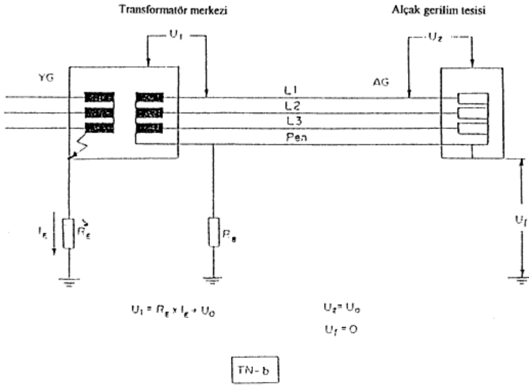
Şekil-9a TN sistemleri
