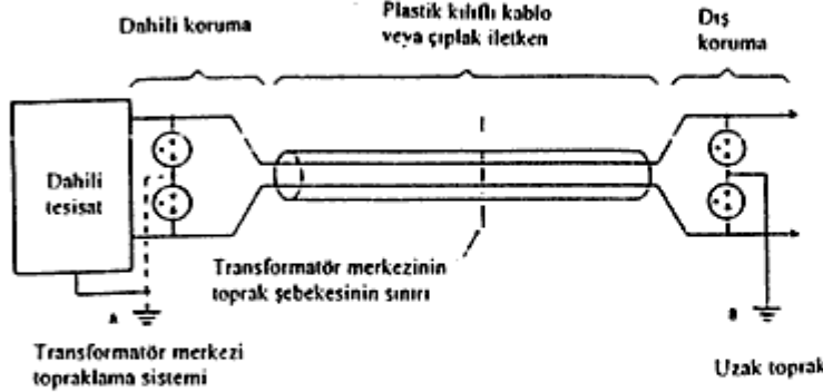
Şekil-Z.1 Koruma için prensip şeması
