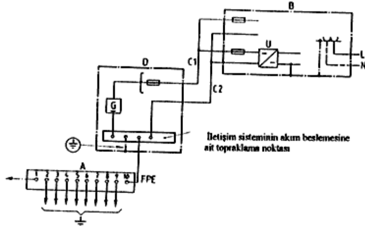
Şekil-14 İletişim sistemine ilişkin akım beslemesinin anma gerilimleri sınırlanmaksızın bir iletişim tesisi için işletme ve koruma topraklamasına örnek (Not: Bu şekil mecburi olmayıp, yalnızca bir fikir vermek amacıyla taşınmıştır.)
