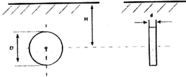
Şekil-T.11 Toprağa düşey olarak gömülen levha topraklayıcı
