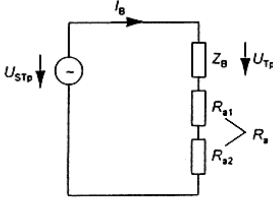
Şekil-C.1 Dokunma devresinin eşdeğer şeması
