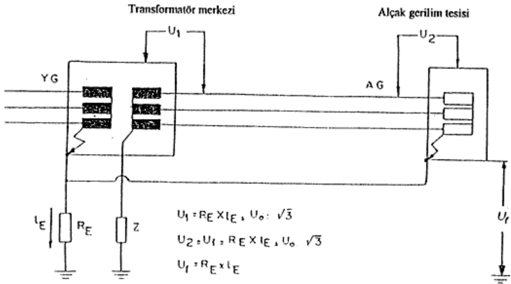
Şekil-9f IT sistemleri, Örnek d
