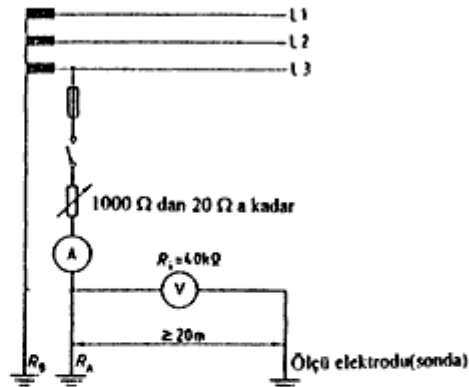
Şekil-8b Topraklama direncinin ölçülmesi için örnek
