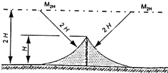
Şekil-II.1 Tek koruma teli
