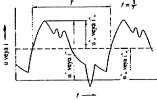
Şekil-Y.2 Doğru bileşeni bulunan, sinüs şeklinde olmayan bir değişim için örnek
