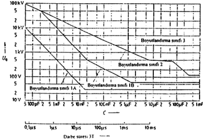
Şekil-12 Farklı boyutlandırma sınıflarında, C kapasitesine bağlı olarak izin verilen dolma (şarj) gerilimleri U_0
